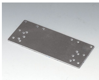
V4116136 Монтажная панель L и M Алюминий матово-анодированный 102x45x1mm
