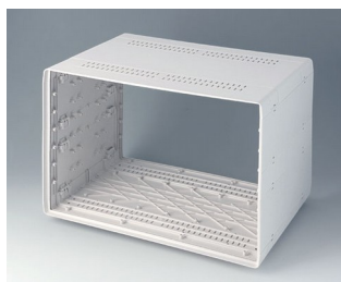
A0266270 EURO CASE 63 HP, без ручки ABC (UL 94 HB) белый RAL 9002 367x250x276,5mm
