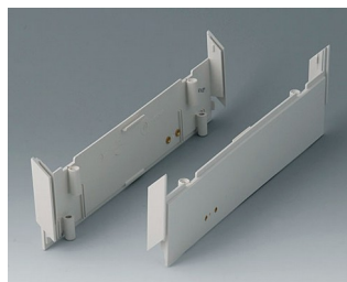
V2030107 Боковые панели 220, с отверстиями для ручки АБС (UL 94 HB) белый RAL 9002
