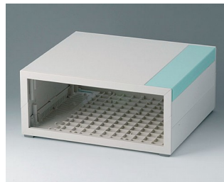
B2210215 MEDITEC D 220, без ручки АБС (UL 94 HB) белый RAL 9002 290x260x124mm IP 40
