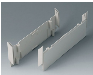
V2030007 Боковые панели 220, без отверстий АБС (UL 94 HB) белый RAL 9002
