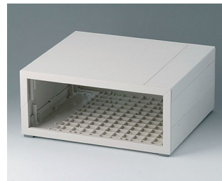
B2210217 MEDITEC D 220, без ручки АБС (UL 94 HB) белый RAL 9002 290x260x124mm IP 40
