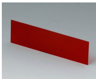
A9108113 Лицевая / задняя панель Акриловое стекло прозр. красная 81,9x23,6x1mm
