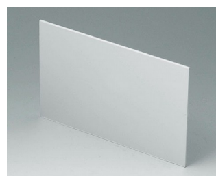
A9114221 Лицевая / задняя панель Алюминий матово-анодированный 124,2x79,6x1,5mm
