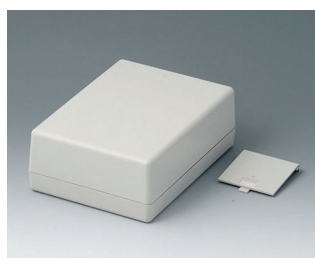
A9413747 SHELL-TYPE CASE G 190, исп. V АБС (UL 94 HB) белый RAL 9002 138x190x68mm
