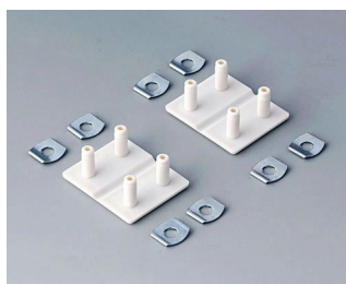
A9193027 Петли ПП белый RAL 9002
