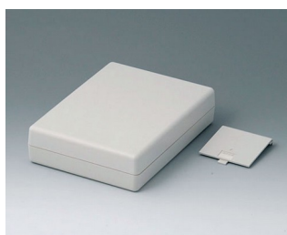
A9413737 SHELL-TYPE CASE G 190, исп. V АБС (UL 94 HB) белый RAL 9002 138x190x45mm
